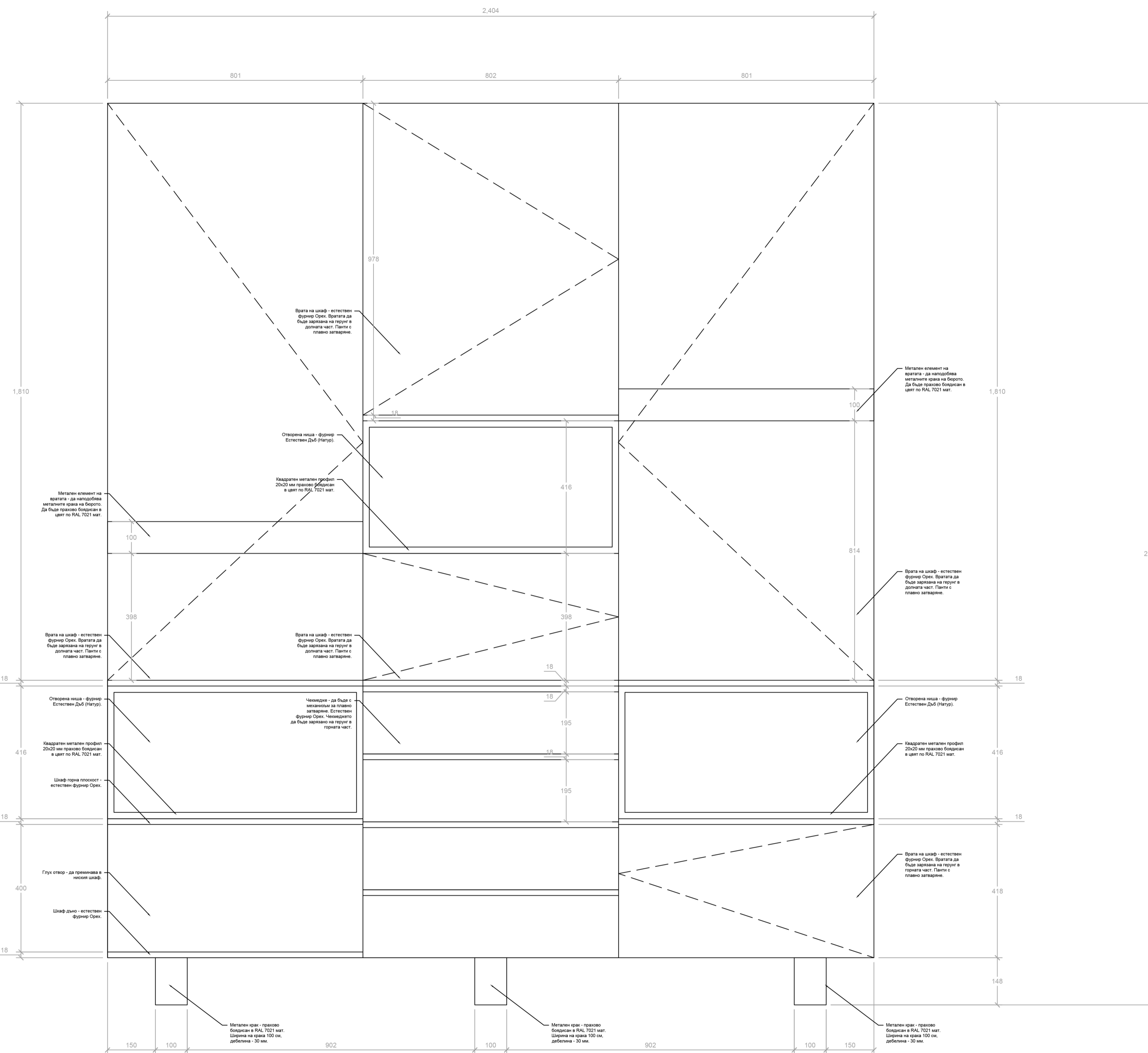
Разгъвка Висок Шкаф Мащаб 1:8
